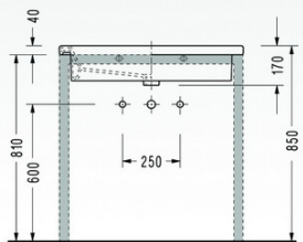
• 8931 Lavabo (tezgaha gömülü)
