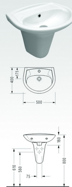
• 2841 Lavabo • 2822 Yarım Ayak
