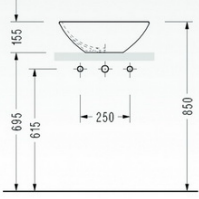
• 2012 Çanak Lavabo Sadece kumandasız bataryalar ile kullanılır.
