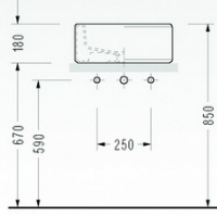
• 2052 Silindirik Lavabo Sadece kumandasız bataryalar ile kullanılır.
