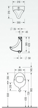
• 0149UZ Pisuar (üstten temiz su çıkışlı)
