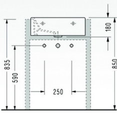
• 2043 Lavabo (yarım tezgah üstü)
