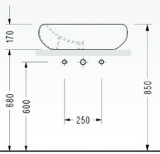
• 7433 Lavabo (tezgah üstü)
