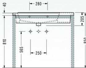
• 8934 Lavabo (tezgaha gömülü)
