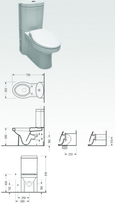
• 6502 BTM Takım Klozeti • 6504 Rezervuar
