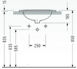
• 1841 Lavabo (tezgah gömülü)
