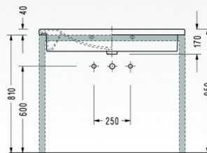
• 8944 Lavabo (tezgaha gömülü)
