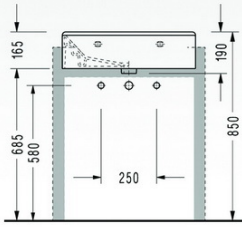
• 2044 Lavabo (yarım tezgah üstü)
